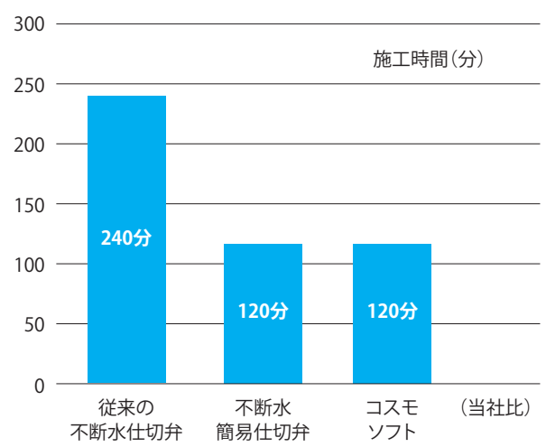
施工時間 比較グラフ φ200の場合
